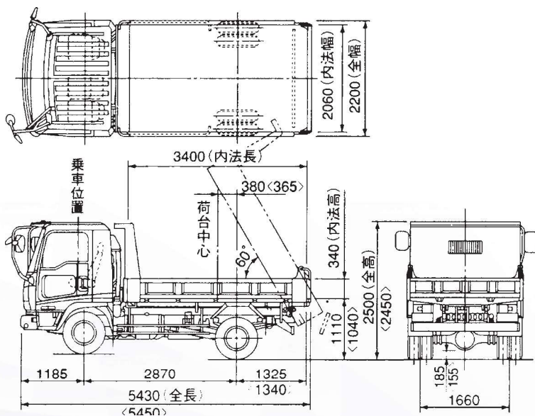
いすず4tダンプ寸法図
