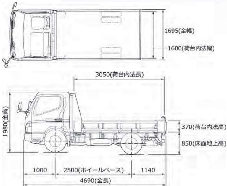
いすず3tダンプ寸法図
