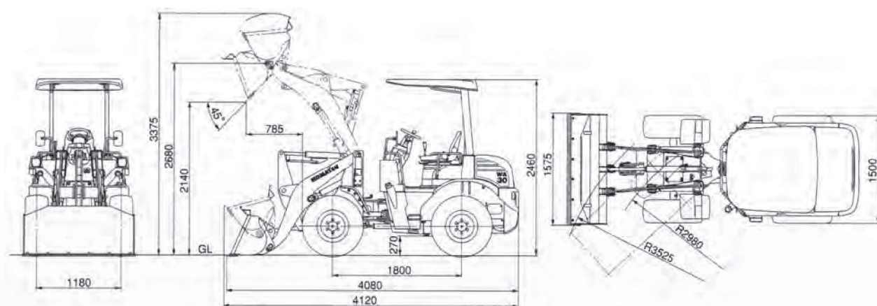
WA40 寸法図
