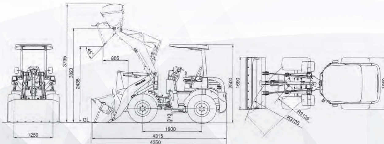
WA40 寸法図
