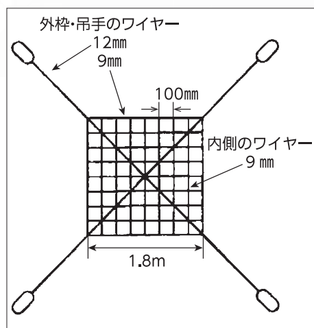
ワイヤーモッコを広げた時の形
