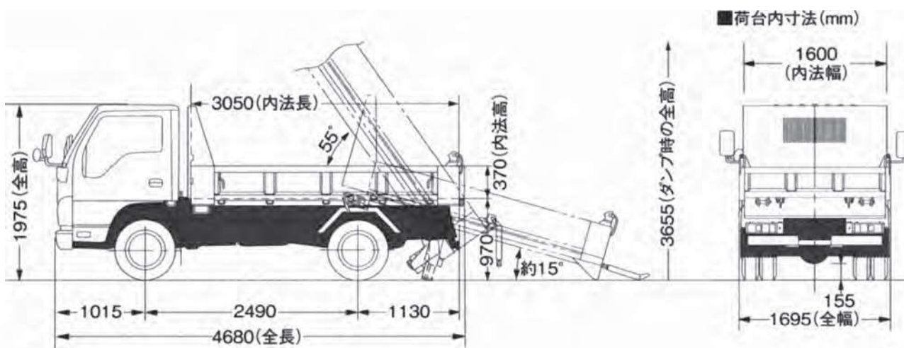
いすゞ寸法図
