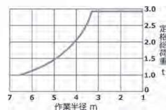
ZX135UR定格荷重表
