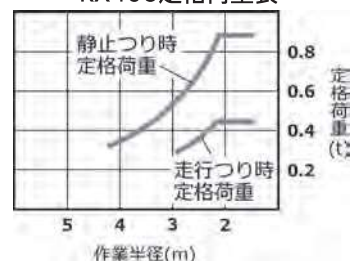
RX406定格荷重表
