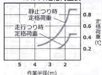
RX306定格荷重表
