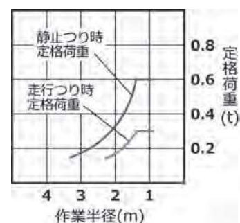
RX203定格荷重表
