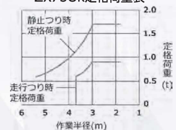
ZX75UR定格荷重表
